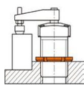
Con tuerca ranurada desde arriba
